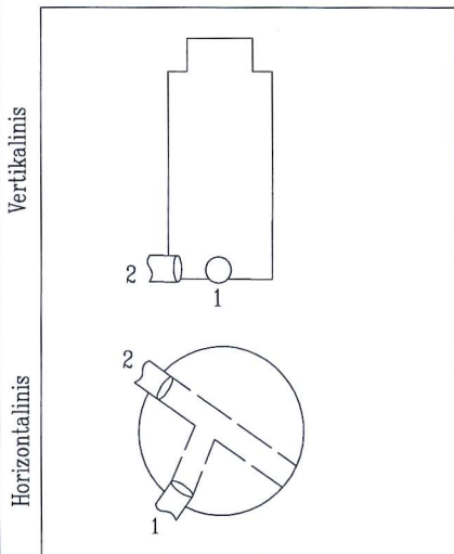
ŠULINIO PĖJŲVAI (Matmenys duokite m)
