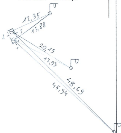
Pririšimo brėžinys
