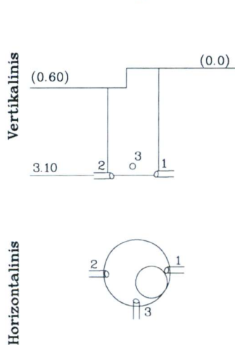
Šulinio pjūviai :
