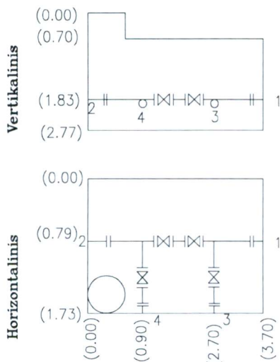
Šulinio pjūviai :
