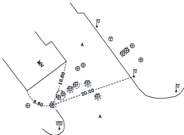
Pririšimo brėžinys
