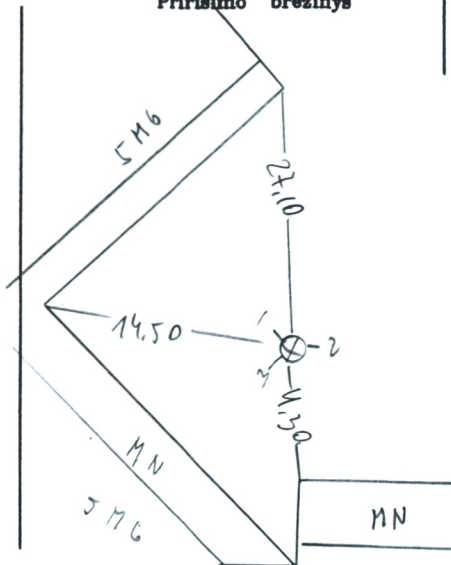
Pririšimo brėžinys
