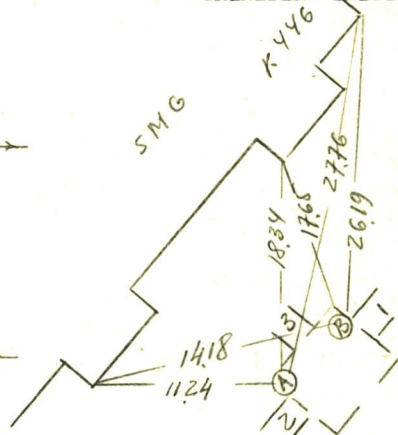
PRIRIŠIMO BRĖŽINYS:
