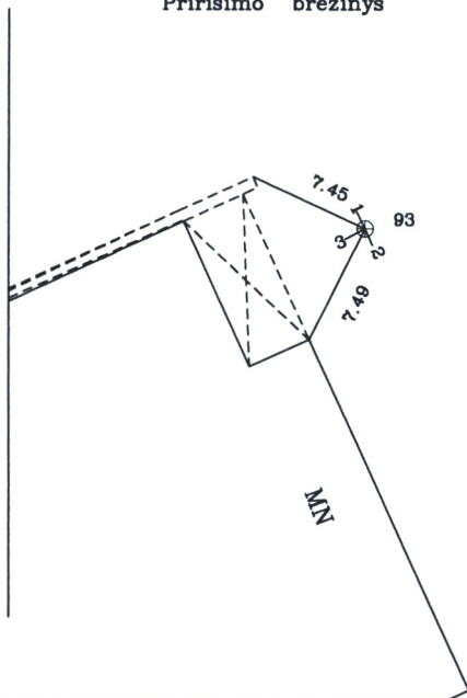
Pririšimo brėžinys
