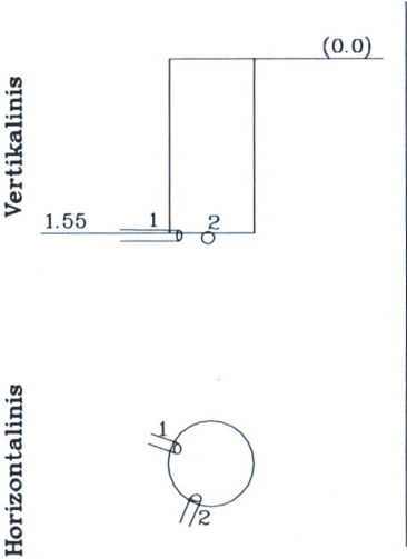
Šulinio pjūviai :
