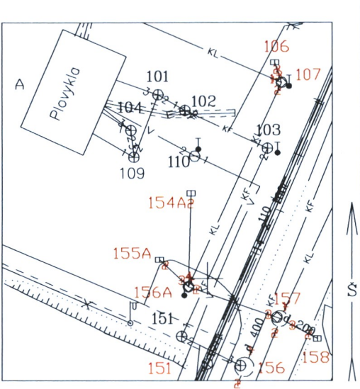
Pririšimo brėžinys :
