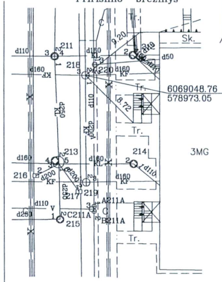
Pririšimo brėžinys
