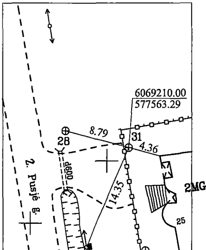
PRIRIŠIMO BRĖŽINYS
