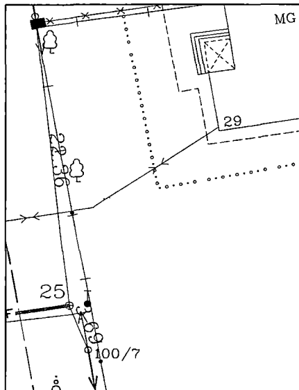
PRIRIŠIMO BRĖŽINYS
