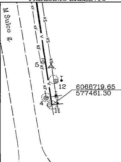
PRIRIŠIMO BRĖŽINYS
