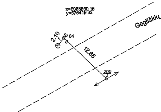
Pririšimo brėžinys
