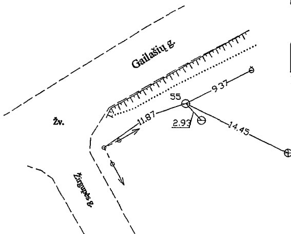
Pririšimo brėžinys
