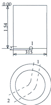
Šulinio pjūviai
