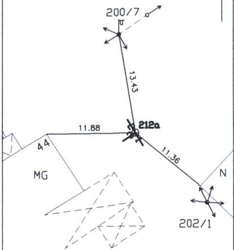
Pririšimo brėžinys
