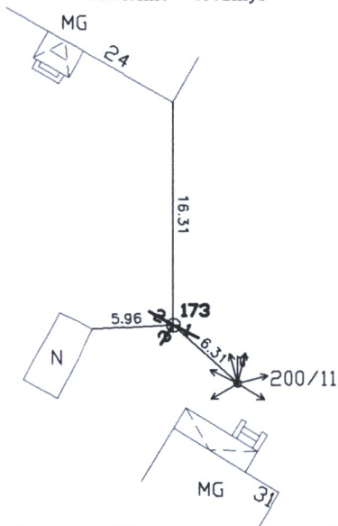
Pririšimo brėžinys
