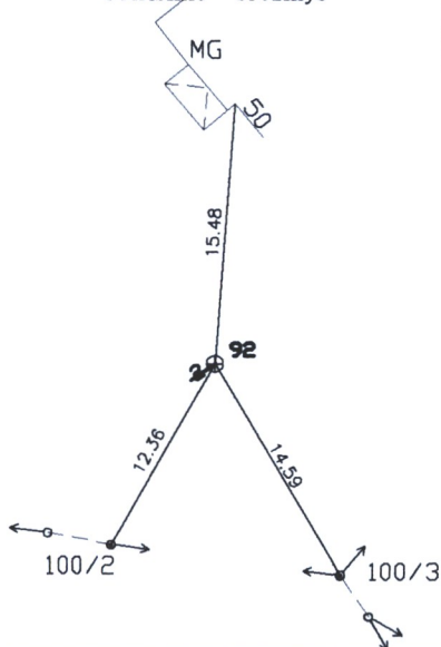
Pririšimo brėžinys
