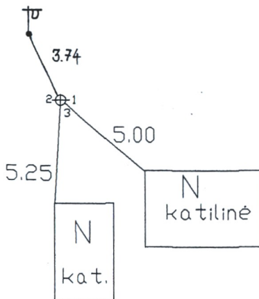
Pririšimo brėžinys
