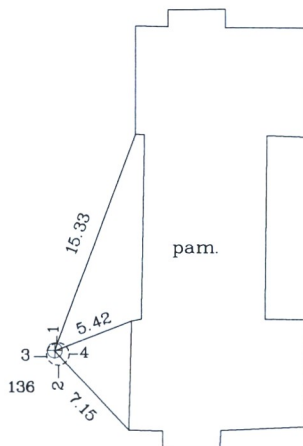
Pririšimo brėžinys
