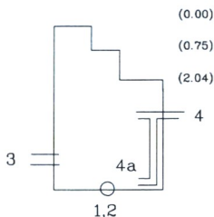
Šulinio pjūviai
