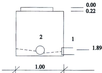
ŠULINIO PJŪVIAI :
