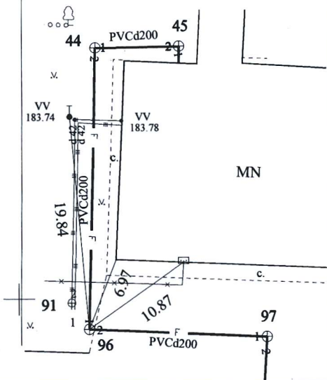
PRIRIŠIMO SCHEMA :
