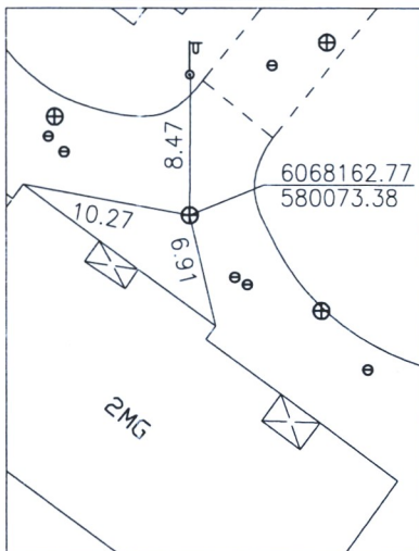
PRIRŠIMO BRĖŽINYS
