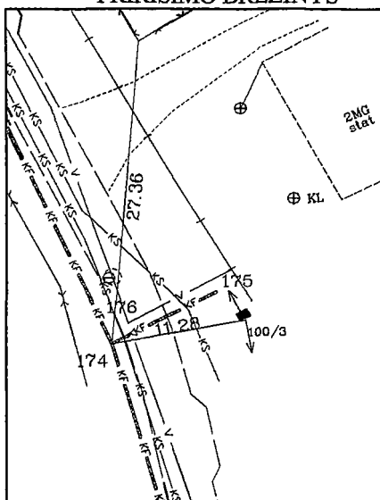
PRIRIŠIMO BRĖŽINYS
