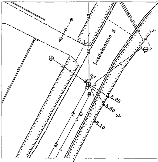
Pririšimo brėžinys
