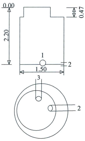
Šulinio pjūviai
