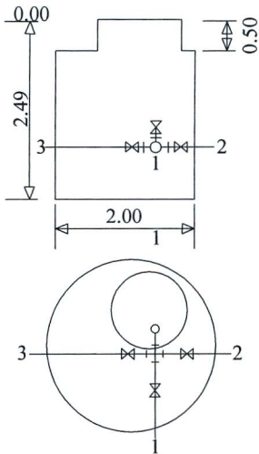
Šulinio pjūviai
