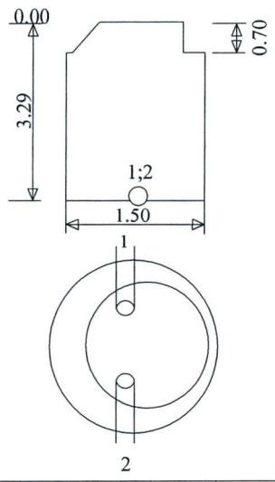
Šulinio pjūviai
