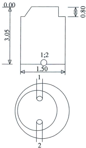
Šulinio pjūviai
