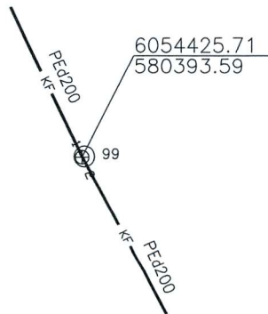
Pririšimo brėžinys
