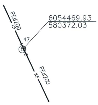
Pririšimo brėžinys
