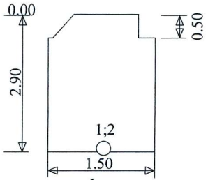
Šulinio pjūviai
