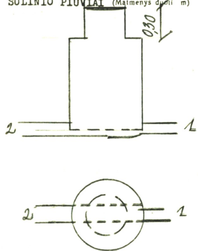
ŠULINIO PLOVIAI (Matmenys duoti m)
