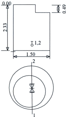
Šulinio pjūviai
