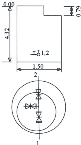
Šulinio pjūviai
