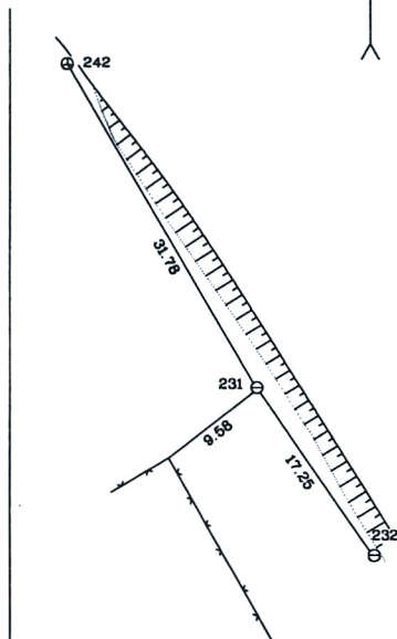
Pririšimo brėžinys
