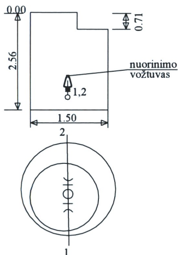
Šulinio pjūviai
