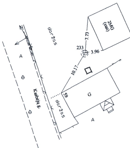
Pririšimo brėžinys
