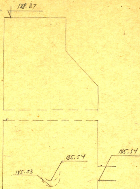
Чертеж колодца М 1:25
