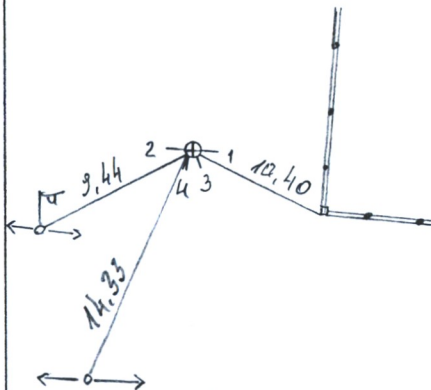
PRIRIŠIMO SCHEMA
