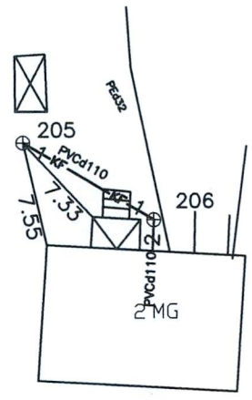
Pririšimo brėžinys
