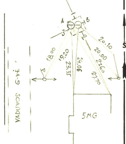
PRIRIŠIMO BRĖŽINYS
