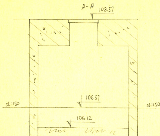
Чертеж колодца М. 1:50
