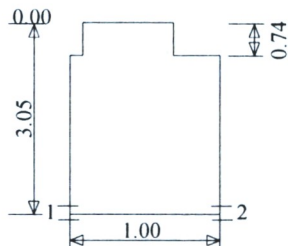
Šulinio pjūviai
