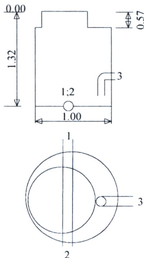
Šulinio pjūviai
