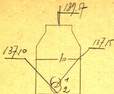
Чертеж колодца М 1:
