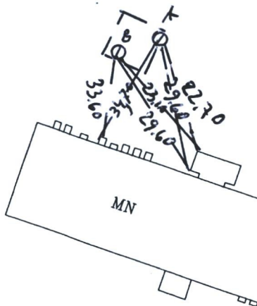
Pririšimo brėžinys
