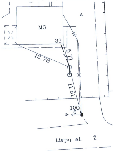
PRIRIŠIMO BRĖŽINYS
