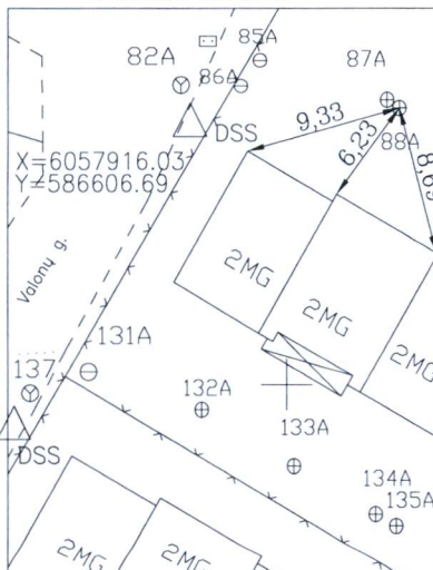
PRIRĖSIMO BRĖŽINYS
