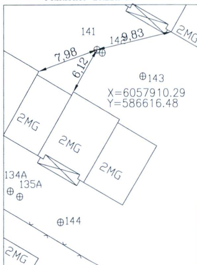
PRIRIŠIMO BRĖŽINYS
