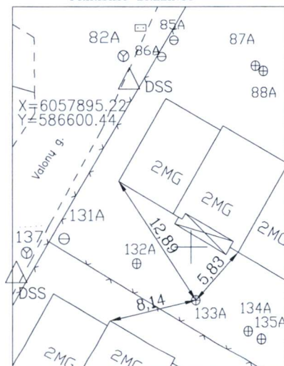
PRIRIŠIMO BRĖŽINYS
